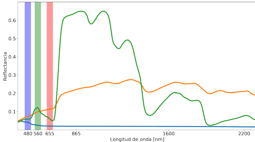
Figura – Interpretación visual - color real.
