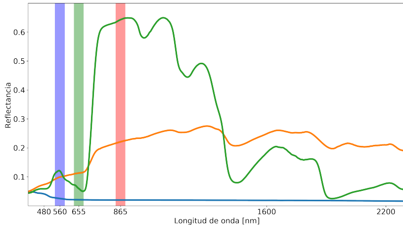
Figura – Interpretación visual - infrarrojo color.
