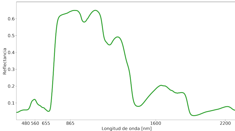
Figura – Firma espectral de la vegetación.
