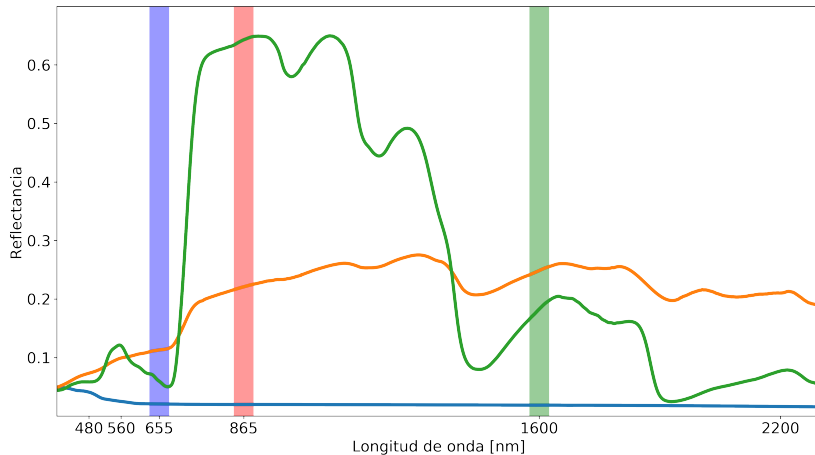
Figura – Interpretación visual - falso color compuesto.
