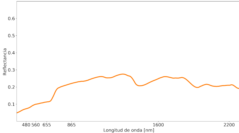
Figura – Firma espectral de la suelo.
